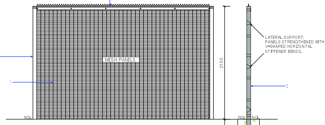
:ELEVATION VIEW :SCALE 1:25
